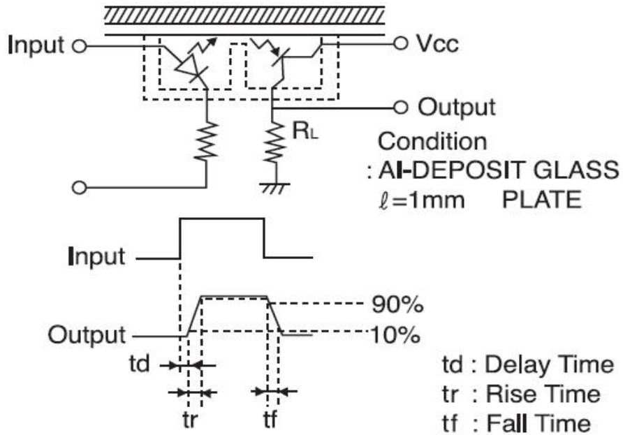
图 3-9 光电传感器上升和下降沿时间测试示意图
