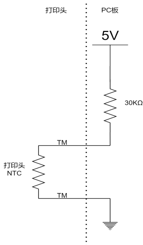
图 3-7 热敏电阻典型电路
