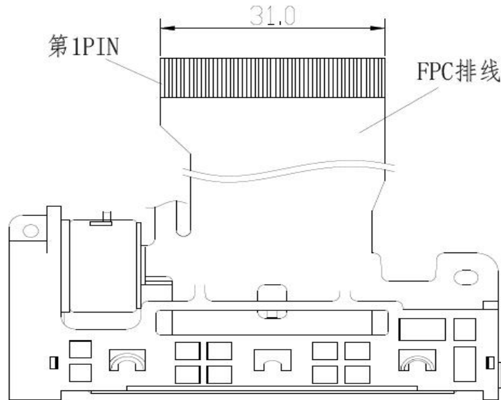
图 4-2 FPC 排线引脚顺序定义图
