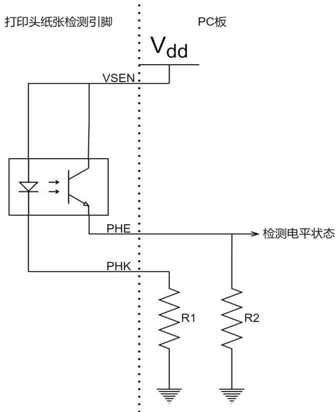
图 3-8 纸张检测电路示意图
