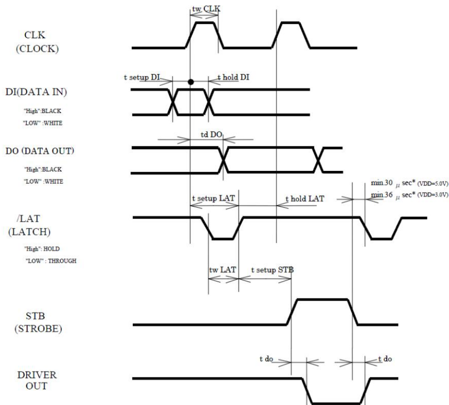
图 3-5 热敏头通信时序图
