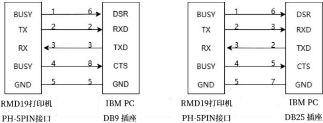
图 3-2 打印机串行接口与 PC 机串行接口连接示意图
