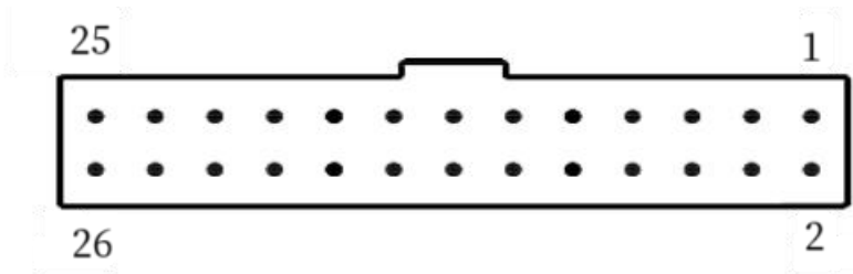
图 3-3 并行接口引脚序号
