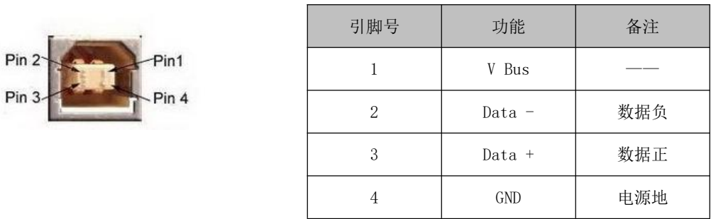
图 3-5 USB 插座及引脚定义
