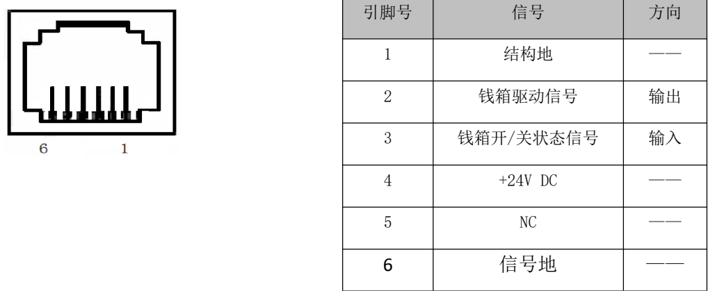
图 3-7 钱箱接口及引脚定义
