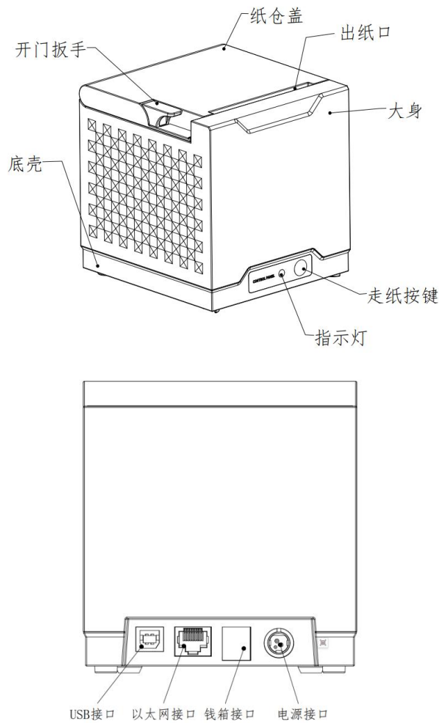
SP-POS895 外观图
