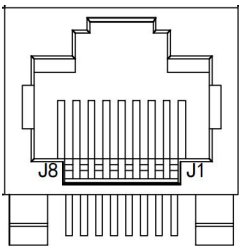
图 3-6 网线接口
